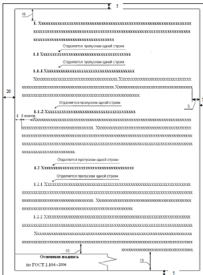
Рисунок 1 — Схема расположения текста и заголовков на листах текстовых учебных документов (размеры указаны в мм)
