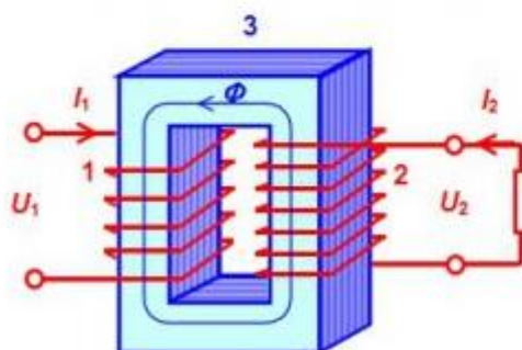
Рисунок 1 – Устройство трансформатора
